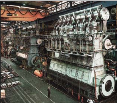
Provkörning - fartygsmotorer
